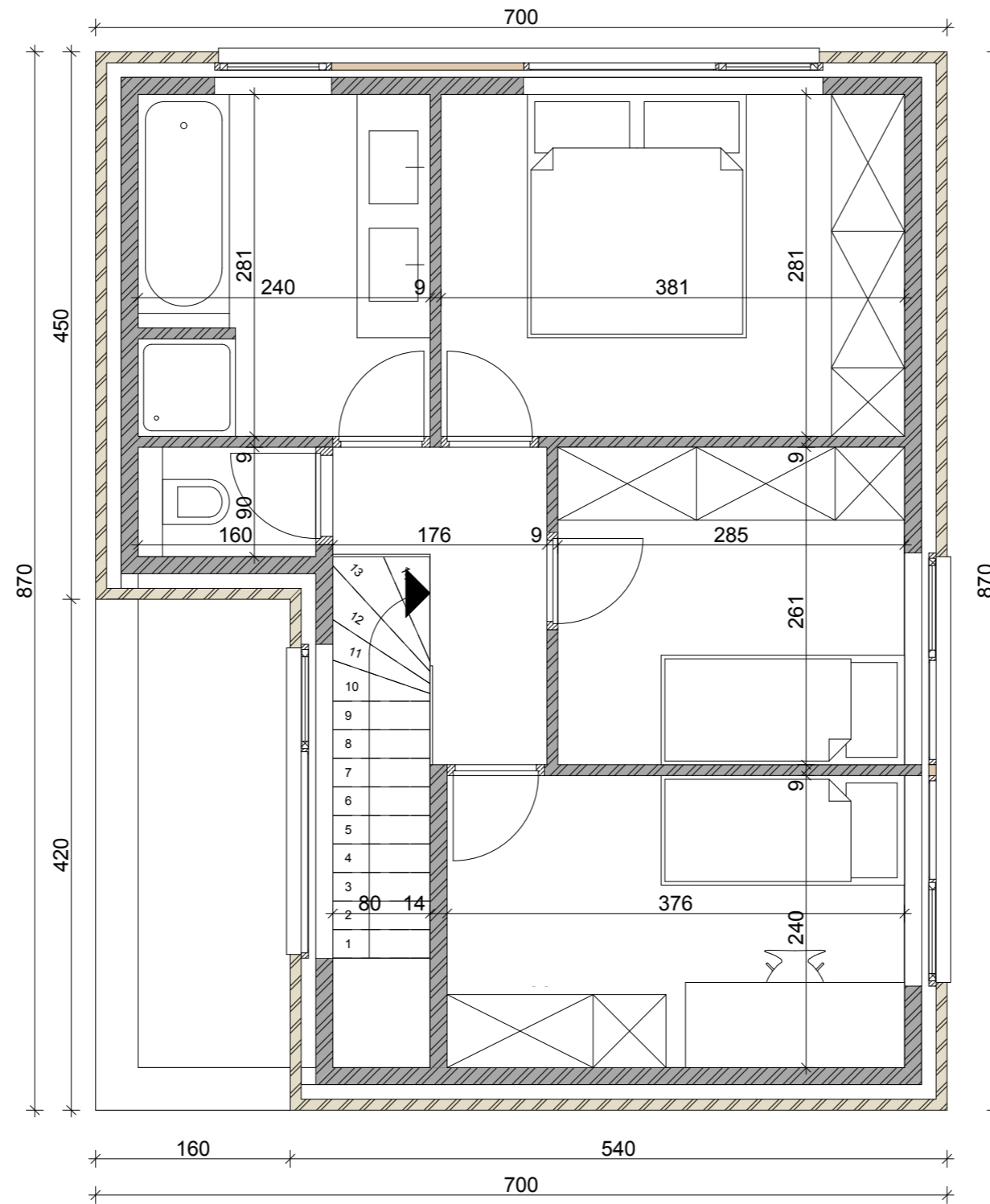
Verdieping
