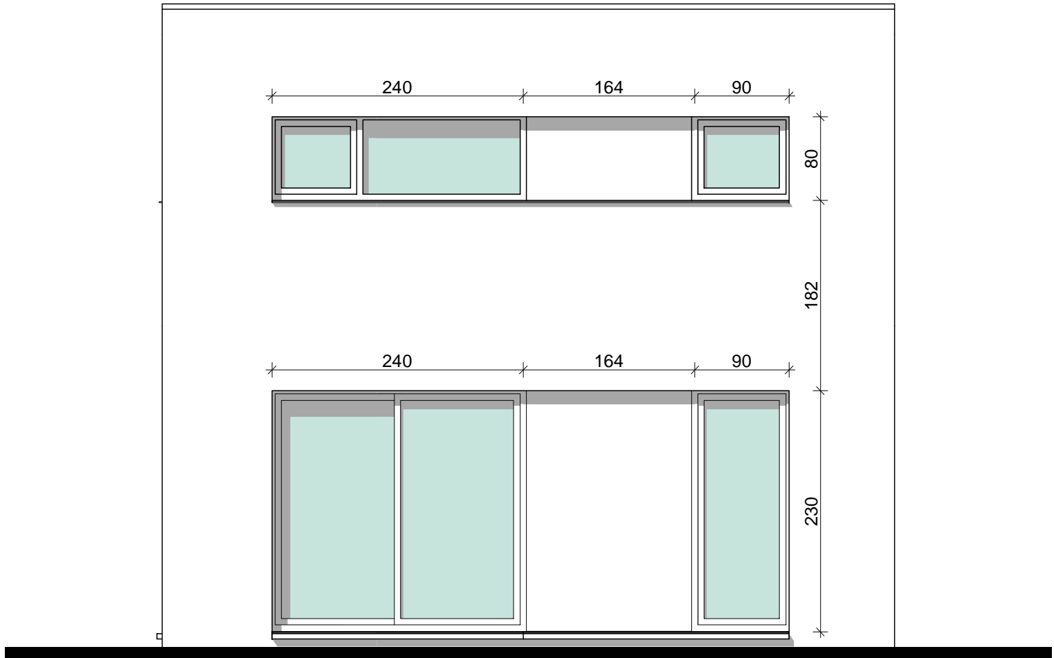
Achtergevel
