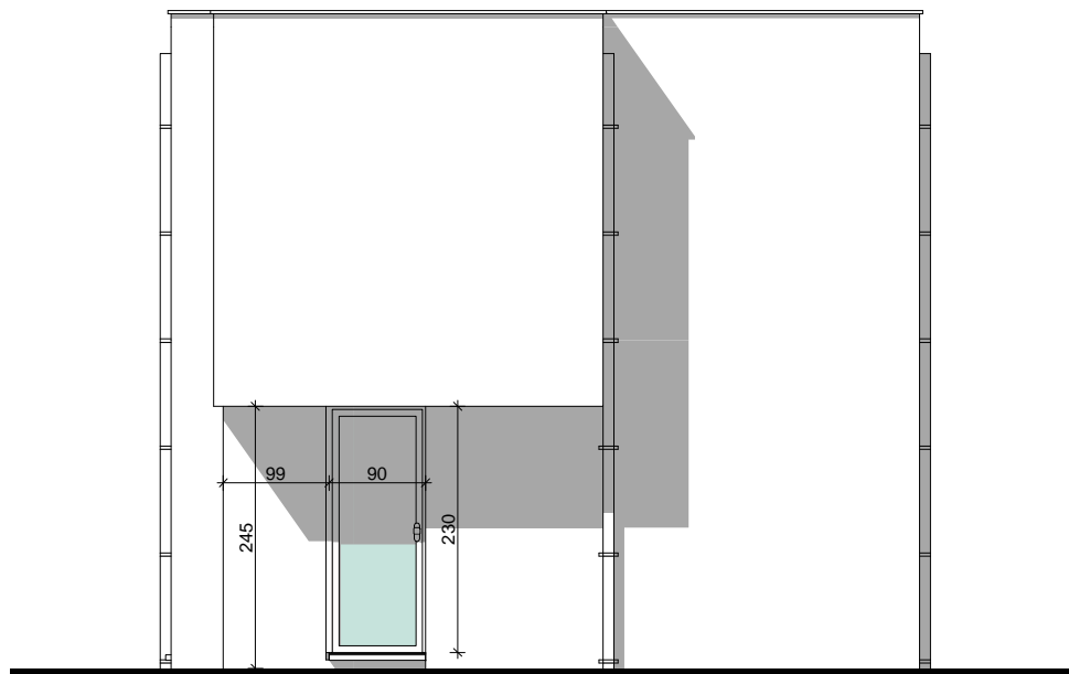
Zijgevel rechts
