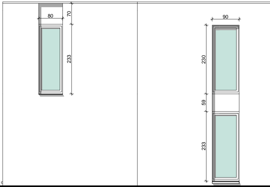
Zijgevel rechts
