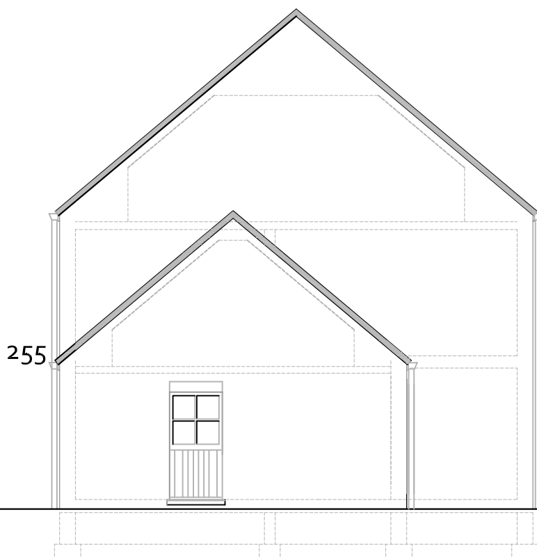
FACADE DROITE
