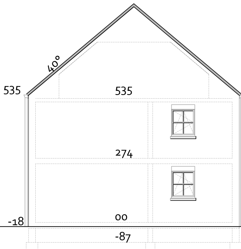
FACADE GAUCHE
